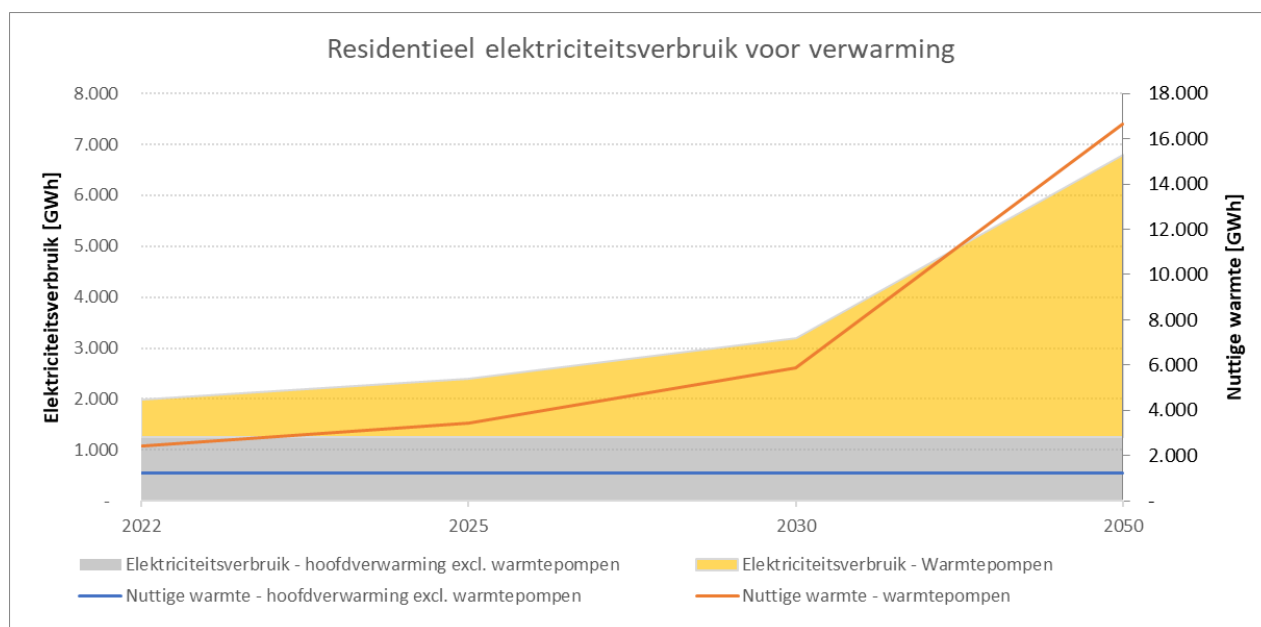
Figuur 2410: Residentieel elektriciteitsverbruik voor verwarming (projectie 2050)
